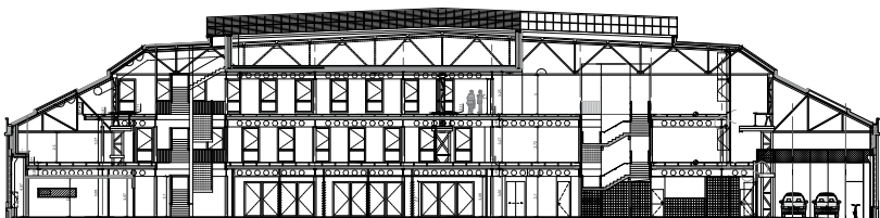
Coupe transversale de la halle.
