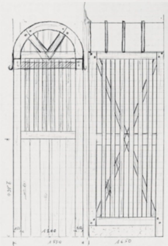
Face et profil de la guérite d'entrée du fort, construction de défense en chêne et toit cintré en cuivre.
