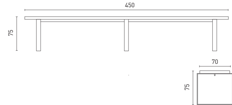
ref. MANU 06 Table de réfectoire formats : 225 x 70 x 75 450 X 70 x 75
