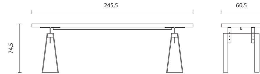
ref. MANU 12 Table d'architecte format : 245,5 x 60,5 x 74,5
